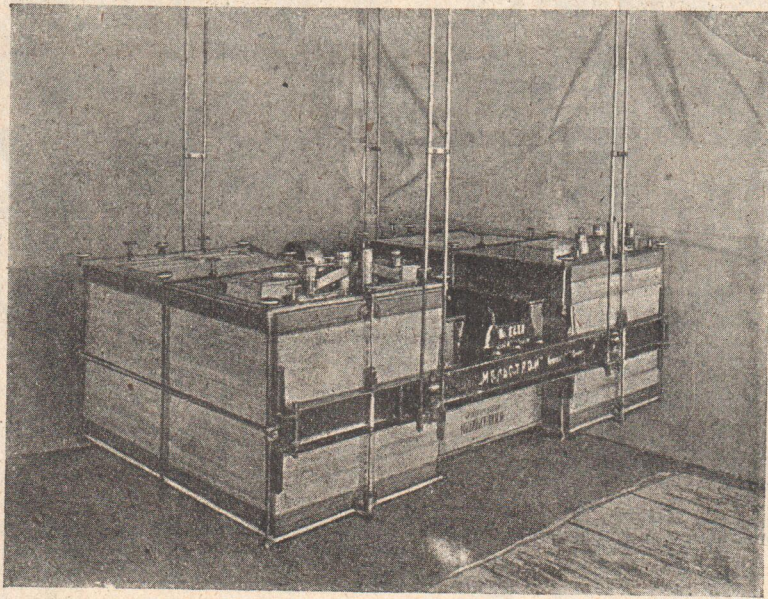
Самобалансирующий бесконечный рассев, — модель 1924 г.
