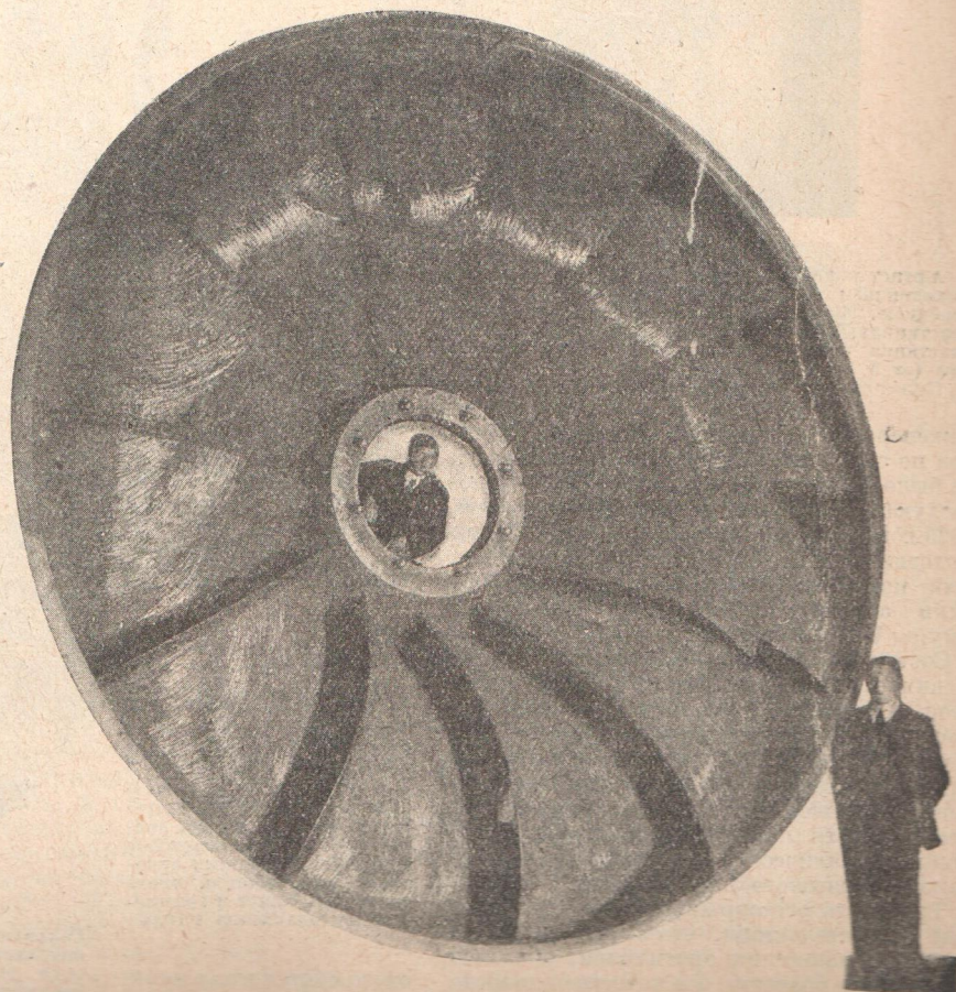
Кососпальная турбина, привезенная из Швеции. У турбины в центре ее шведские инженеры, установившие ее на Волховской гидро-электростанции.
