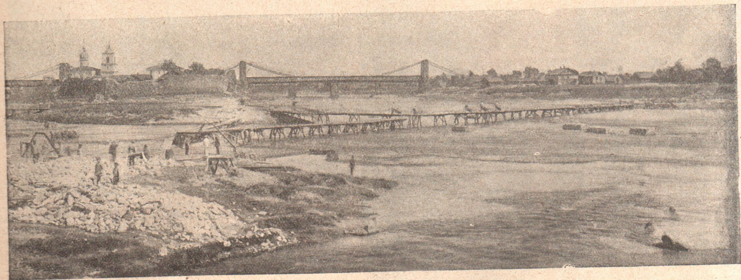
Общий вид работ на плотине гидро-электрической станции на реке Великой.
