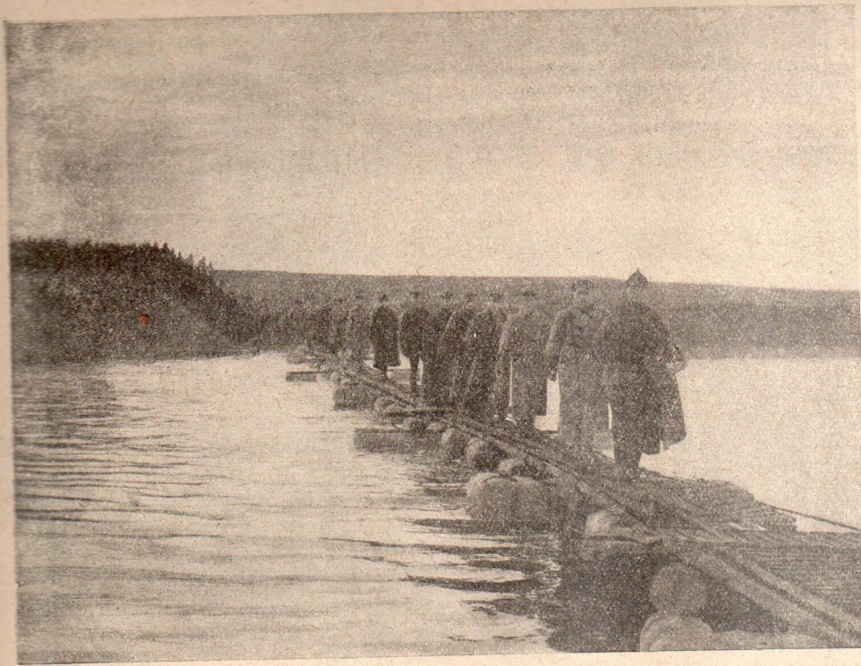
Наводка моста на поплавах системы «Полянского» через реку Коростель в гор. Ярославле.
