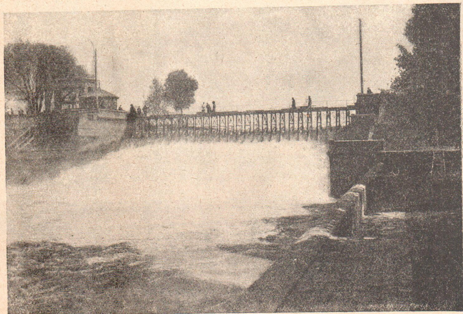
Одна из лучших плотин Туркестана — Гиндукуизская на реке Мургабе в Мервском уезде Туркменской области. При плотине — гидростанция, при помощи которой электрифицирован хлопковый район в Туркменской области — Байрам Амшійский.
